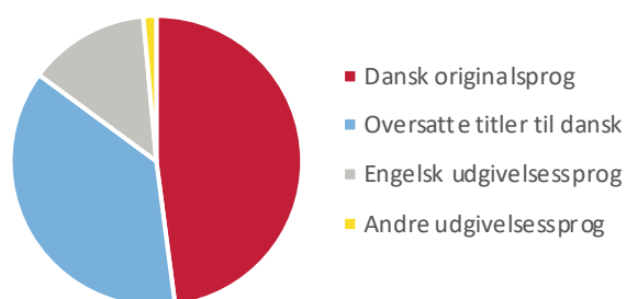
FIGUR 13. BOGSALGET EFTER SPROG I 2023
